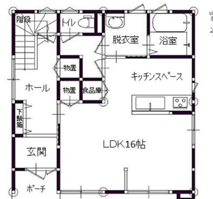
1階平面図
